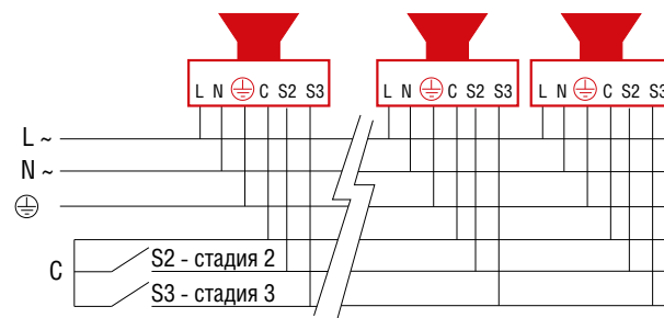
СХЕМА ПОДКЛЮЧЕНИЯ ДЛЯ ПЕРЕМЕННОГО НАПЯЖЕНИЯ
