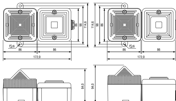
• SONFL1X-HO компактное комбинированное устройство сирена-маяк (с установочными петлями)
