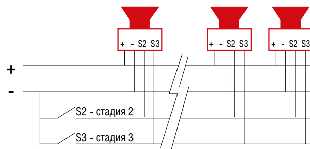
СХЕМА ПОДКЛЮЧЕНИЯ ДЛЯ ПОСТОЯННОГО НАПЯЖЕНИЯ
