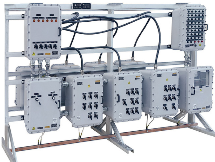
Собранное готовое устройство серии МС 200, состоящее из 11 изделий и смонтированное на единой раме
