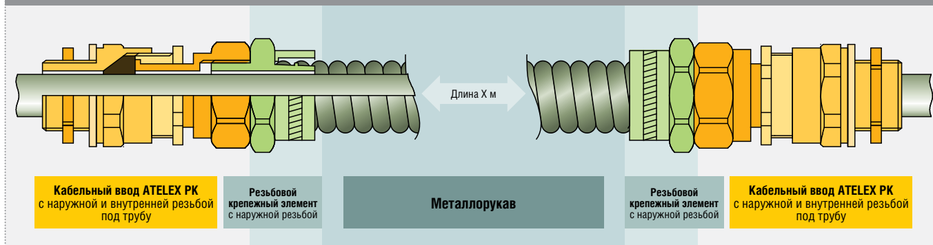
Типовое соединение гибкого металлорукава «Кабельный ввод – Крепежный элемент – Металлорукав – Крепежный элемент – Кабельный ввод»
