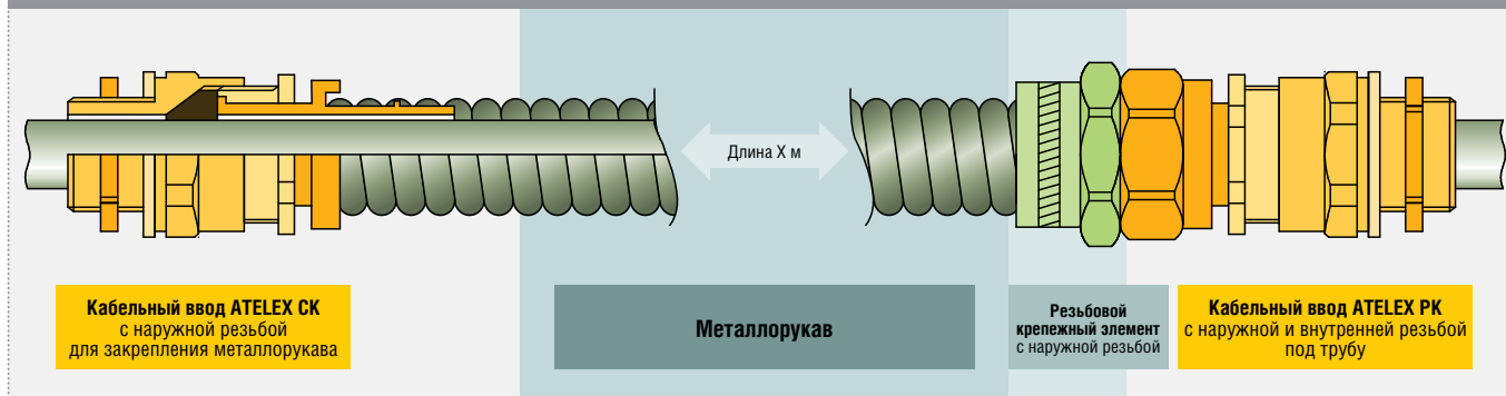
Типовое соединение для закрепления гибкого металлорукава «Кабельный ввод – Металлорукав – Крепежный элемент – Кабельный ввод»
