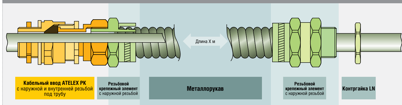
Типовое соединение гибкого металлорукава «Кабельный ввод – Крепежный элемент – Металлорукав – Крепежный элемент – Контргайка»
