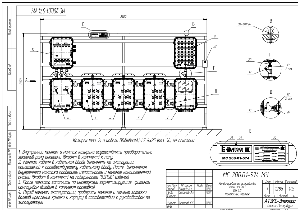
Утвержденный монтажный чертеж MC 200
