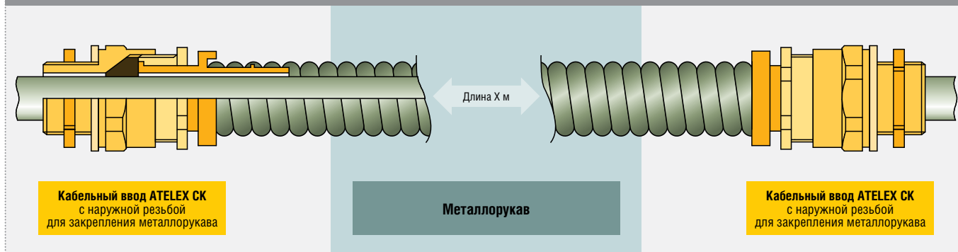
Типовое соединение для закрепления гибкого металлорукава «Кабельный ввод – Металлорукав – Кабельный ввод»
