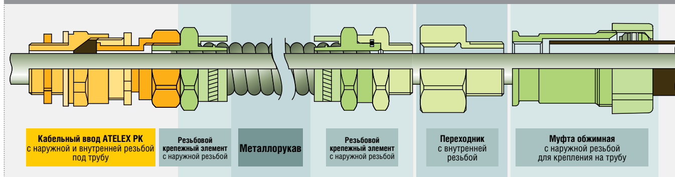
Типовое соединение для закрепления гибкого металлорукава с дальнейшим присоединением на трубу
